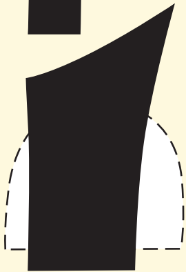
Form 983 Mittlere Höhe 70 mm Hintere Höhe 77 mm Fersenbett-Breite 50 mm
