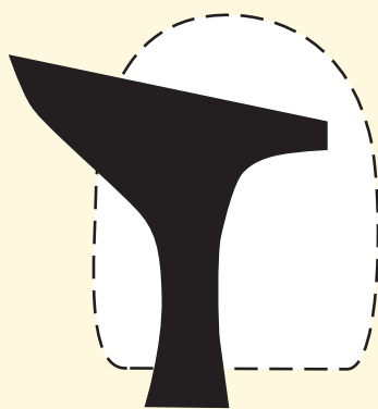
Form 2950 Mittlere Höhe 51 mm Hintere Höhe 60 mm Fersenbett-Breite 49 mm
