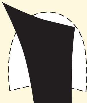
Form 2005 Mittlere Höhe 58 mm Hintere Höhe 66 mm Fersenbett-Breite 48 mm
