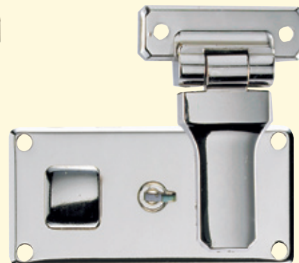
Aktenkofferschloss ca. 65 x 30 mm
