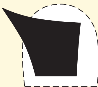
Form 2001 Mittlere Höhe 42 mm Hintere Höhe 48 mm Fersenbett-Breite 50 mm
