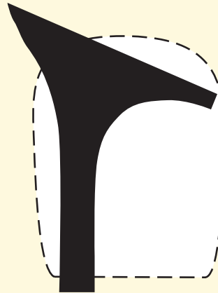
Form 2980 Mittlere Höhe 70 mm Hintere Höhe 77 mm Fersenbett-Breite 50 mm
