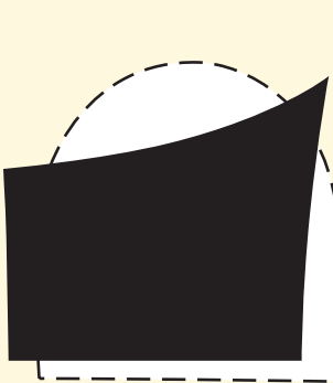
Form 44 Mittlere Höhe 44 mm Hintere Höhe 49 mm Fersenbett-Breite 55 mm
