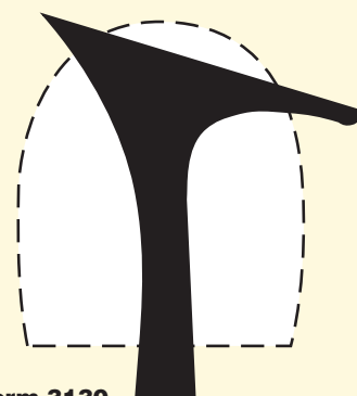
Form 3130 Mittlere Höhe 60 mm Hintere Höhe 66 mm Fersenbett-Breite 50 mm
