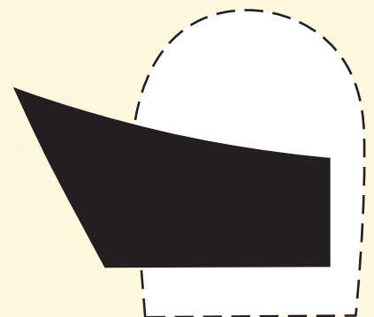
Form 752 Mittlere Höhe 33 mm Hintere Höhe 37 mm Fersenbett-Breite 50 mm
